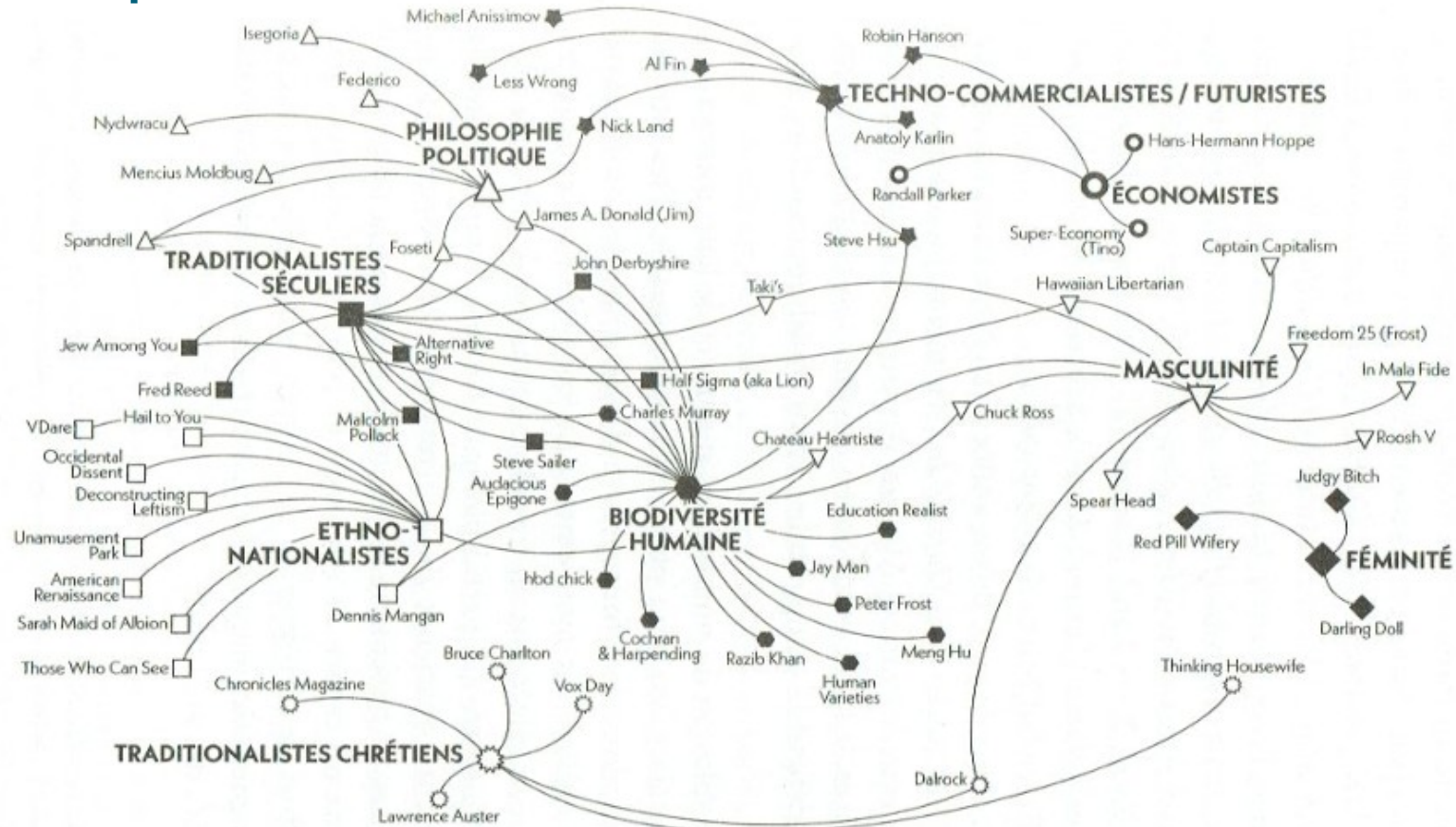
Figure 2 : Cartographie de la droite numérique par Scharlach (Habitable Worlds)
