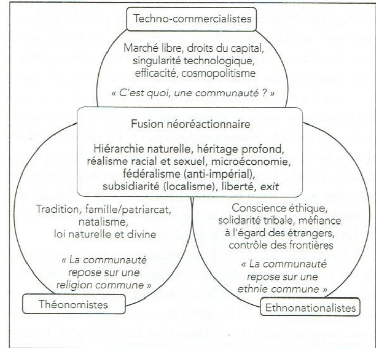
Figure 3 : La trichotomie de Spandrell, reprise par Nick B. Steves (adap-
